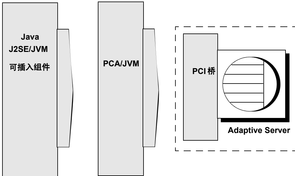
图 2-1: Java 组件
