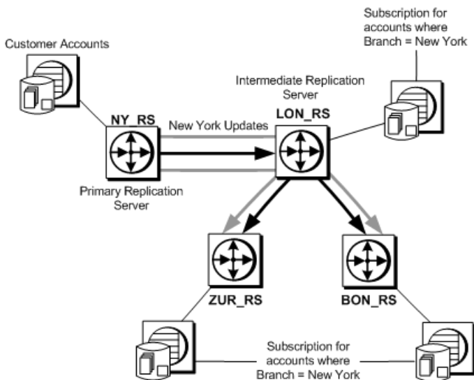
图 12：具有重叠预订的节点
