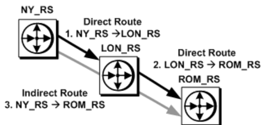
图 14：创建直接路由和间接路由的顺序
