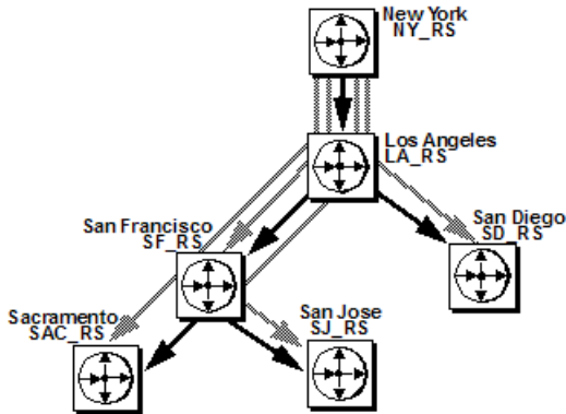
图 17: 更改后的间接路由
