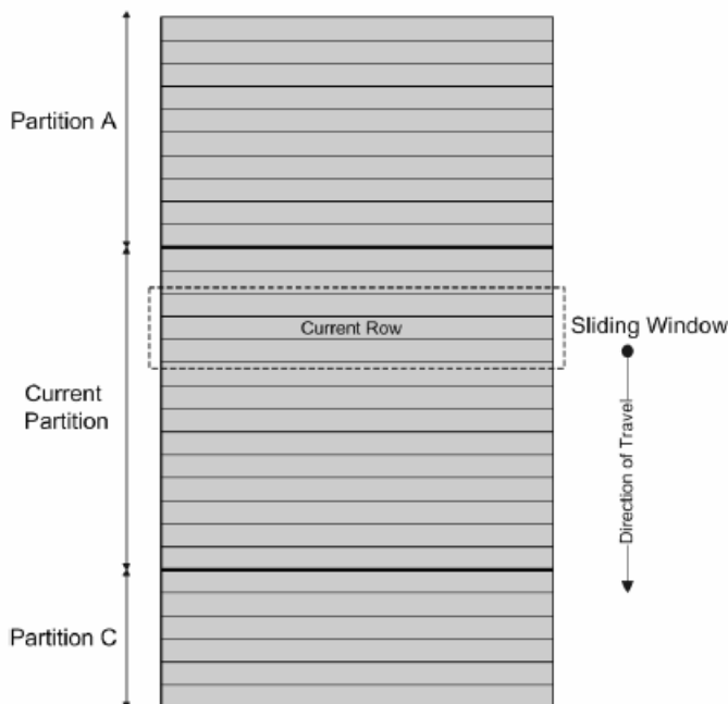
图 3：含分区输入的三行移动窗口
