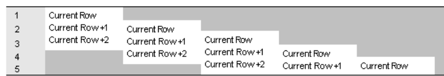
图 4：基于行的窗口构架
