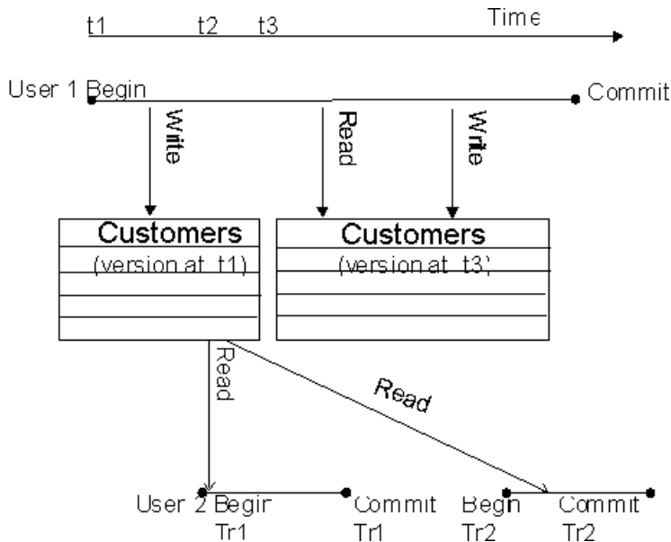
図 5：トランザクションによるコミットされたデータの使用
