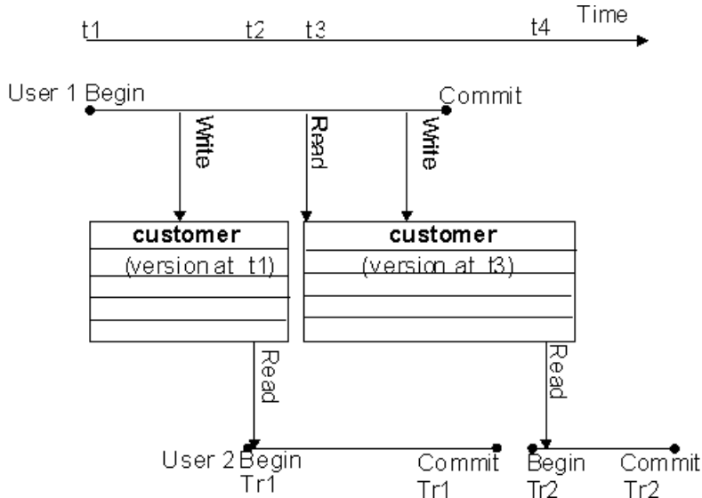
図 6 : 読み取りトランザクションのコミットの影響
