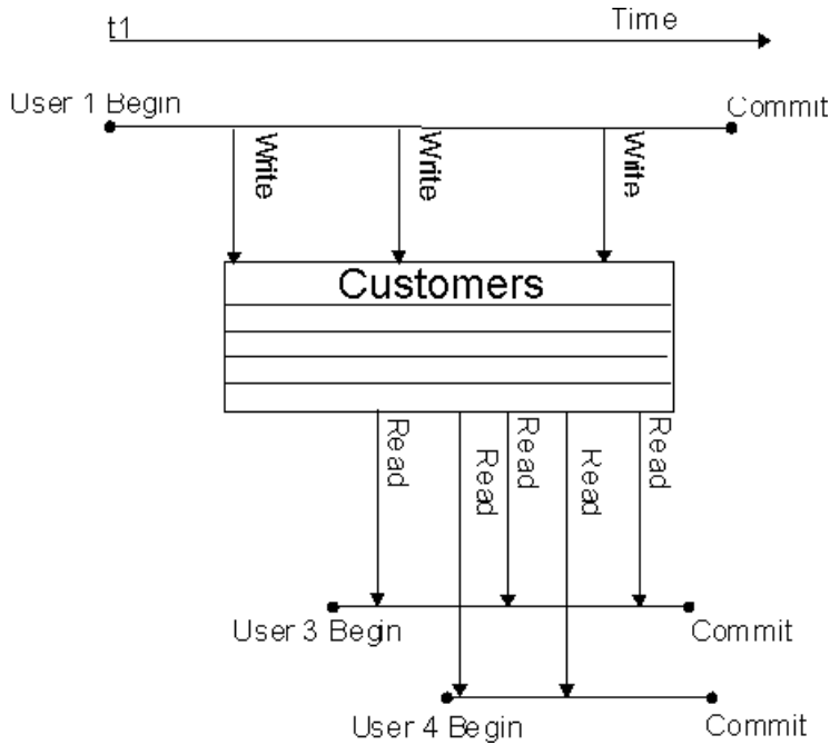
図 3 : 1 人の書き込みユーザ、複数の読み取りユーザ
