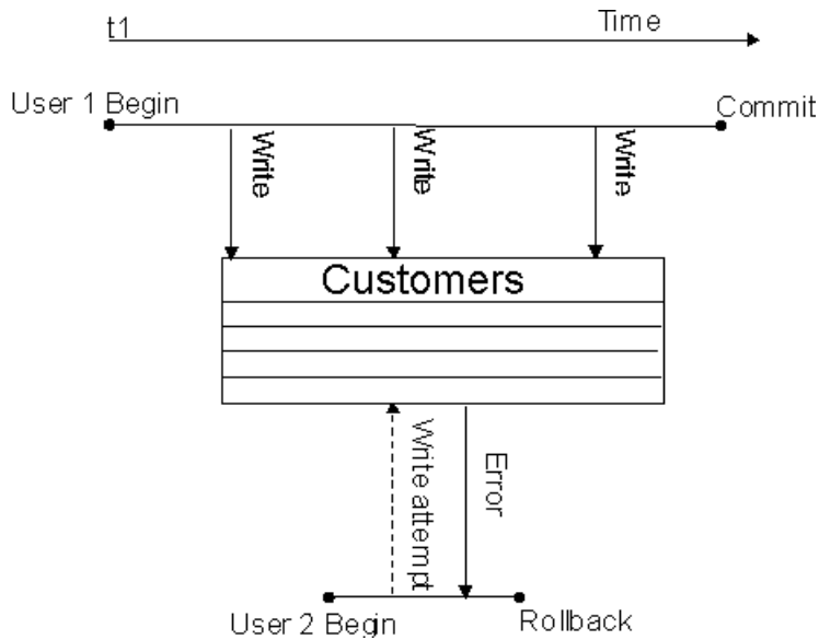
図 2：一度に 1 人の書き込みユーザ
