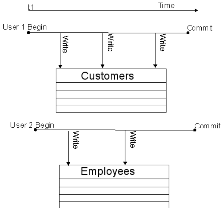
図 4 : 異なるテーブルへの同時挿入
