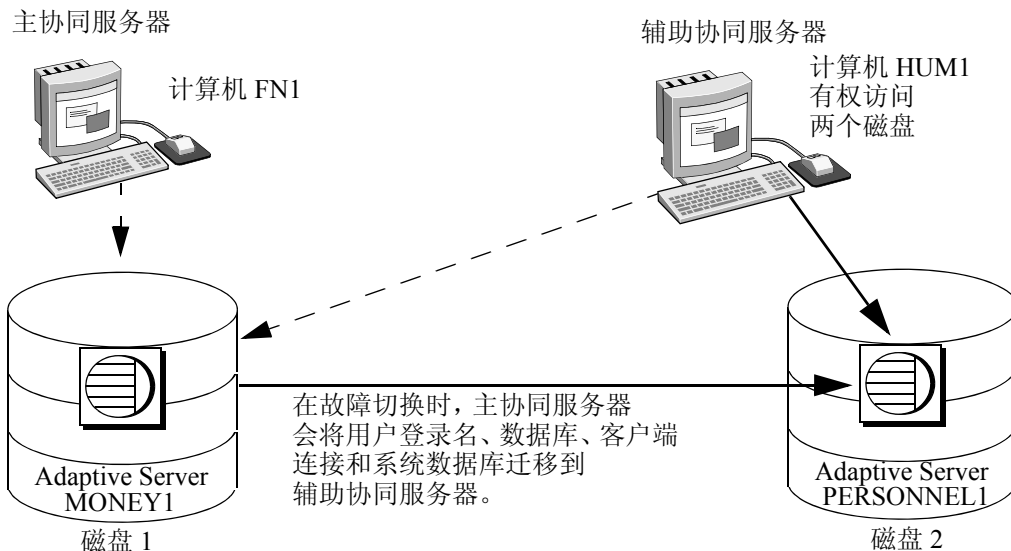
图 3-1：高可用性系统中的非对称配置
