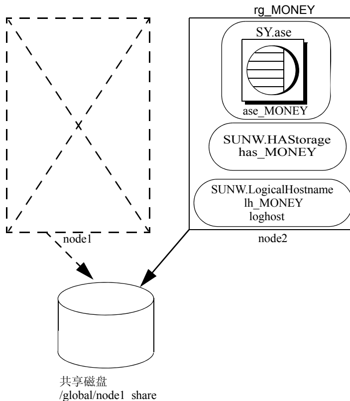
图 10-2: 故障切换后 Sun Cluster 上的主动 - 被动式设置
