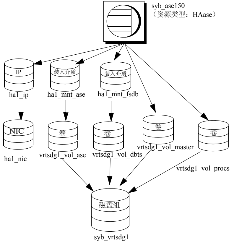
图 11-1: 在 Veritas Cluster Server 上运行的样本服务组
