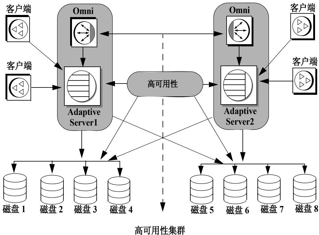
图 2-1: 使用 Sybase 故障切换的高可用性系统
