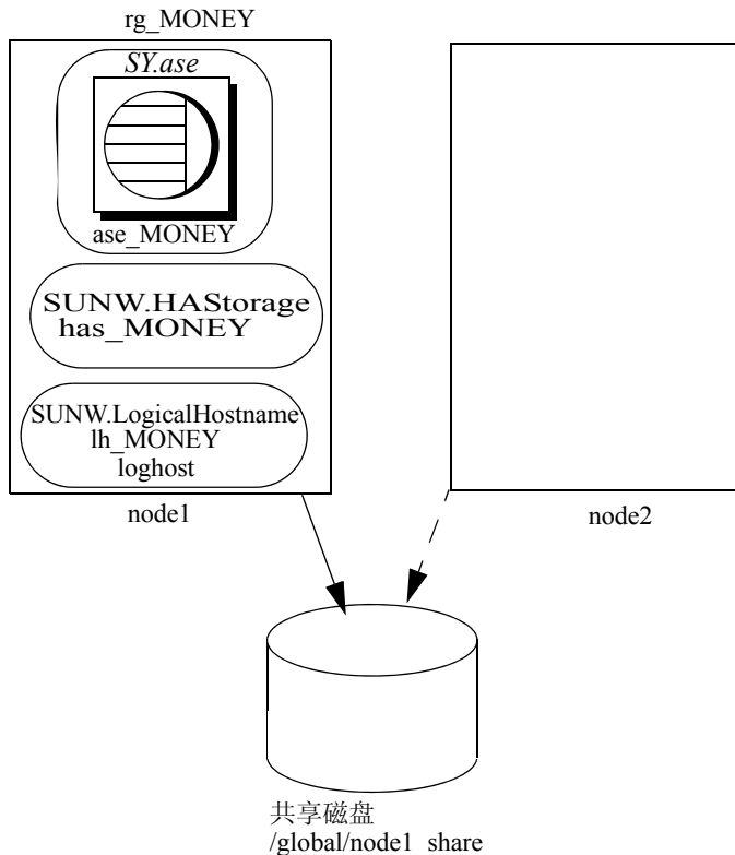
图 10-1: 故障切换前 Sun Cluster 中的主动 - 被动式设置
