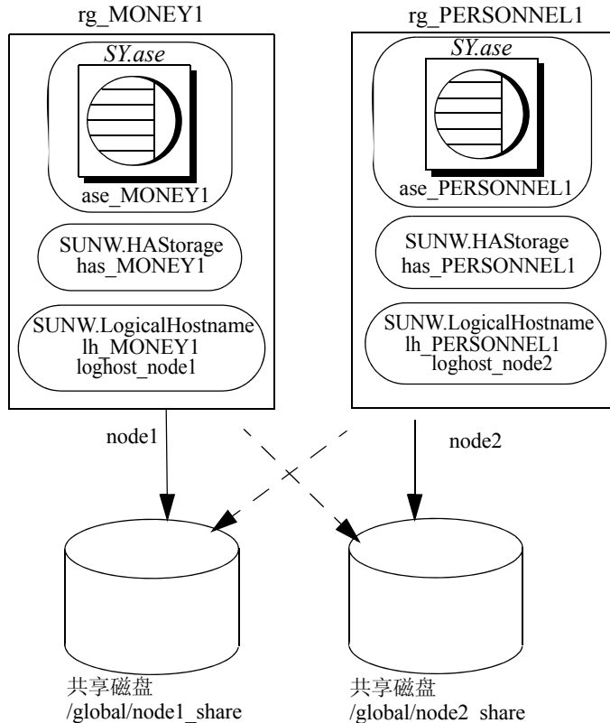
图 9-1: Sun Cluster 资源组配置示例
