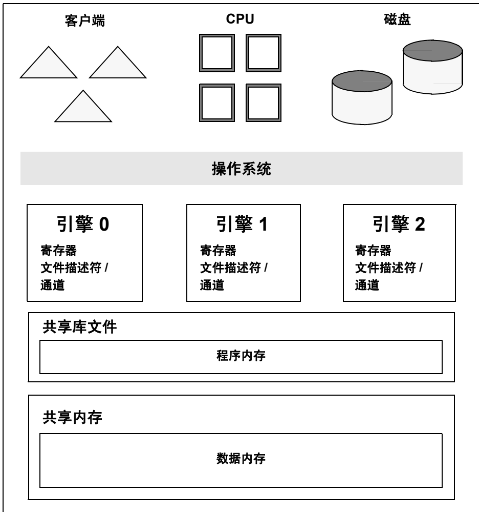
图 5-1: SMP 环境体系结构
