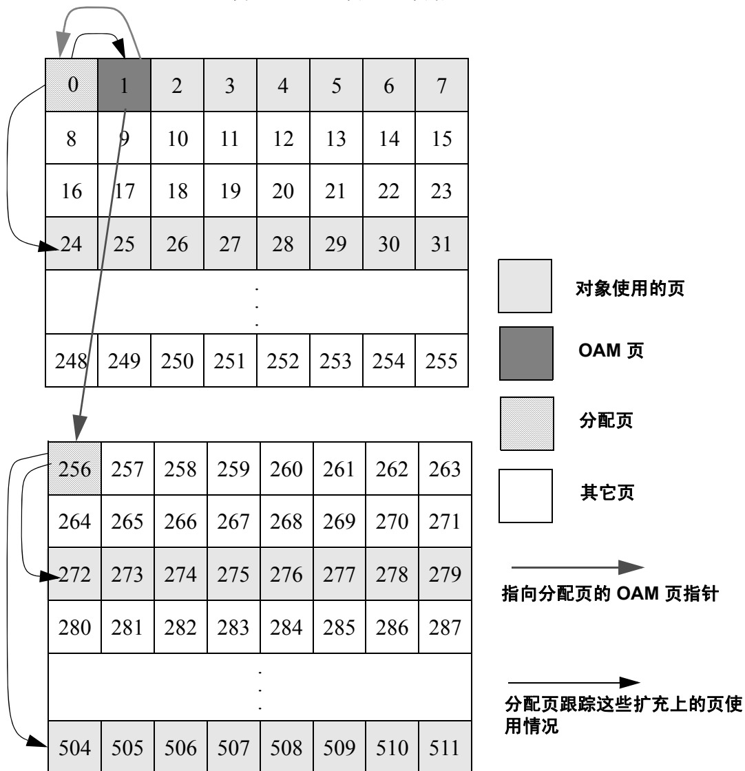
图 10-2: OAM 页和分配页指针
