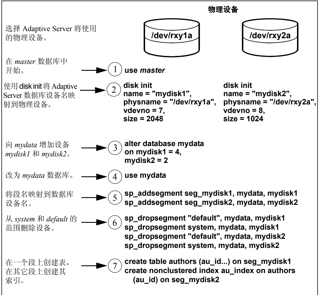
图 8-3: 使用段在特定设备上创建对象
