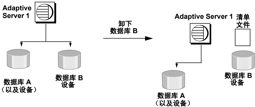
图 7-1: unmount 命令
