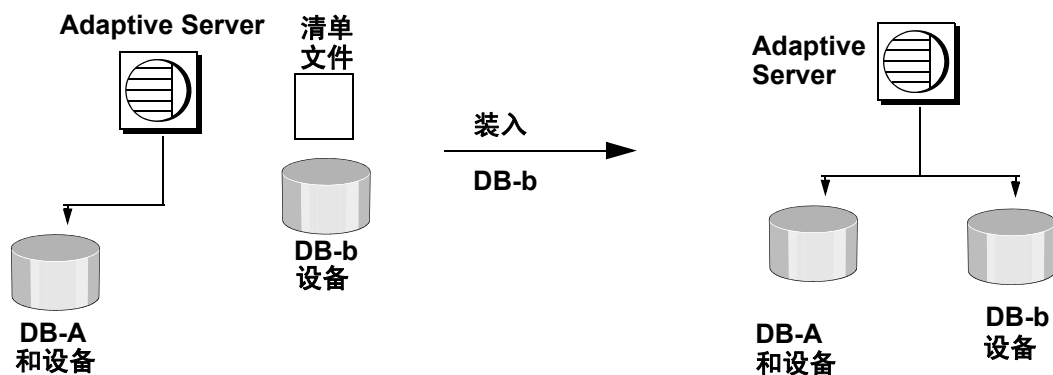
图 7-2: mount 命令
