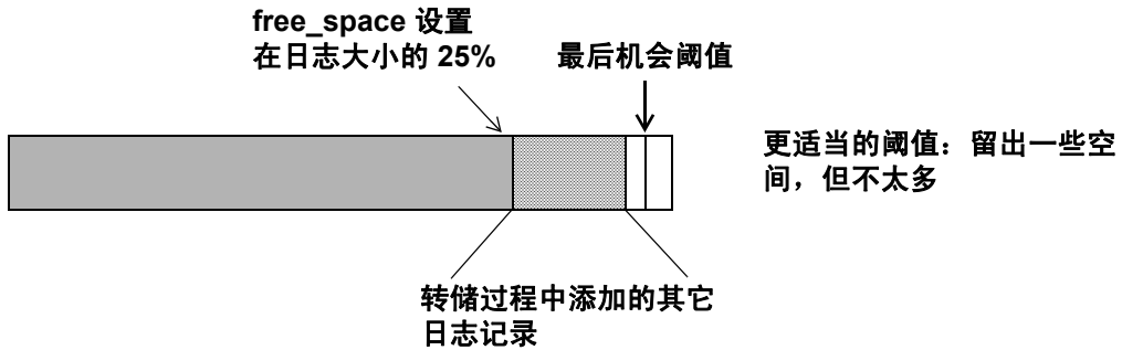
图 16-7: 移动阈值使转储后留下较少的可用空间
