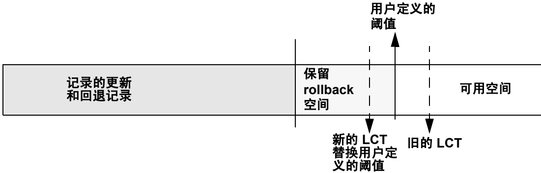
图 16-4: 在达到用户定义的阈值之前引发 LCT
