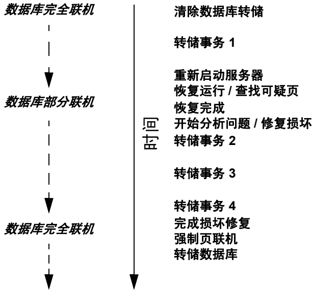
图 11-2: 修复策略
