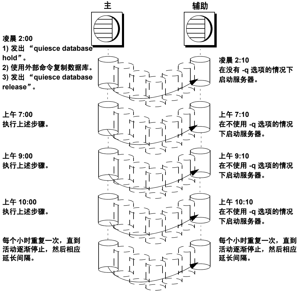
图 11-6: 迭代刷新方法的备份安排
