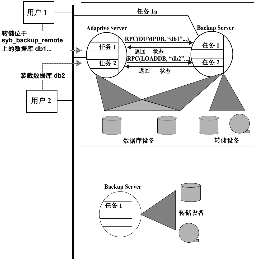
图 11-8: Adaptive Server 与具有远程 Backup Server 的 Backup Server
