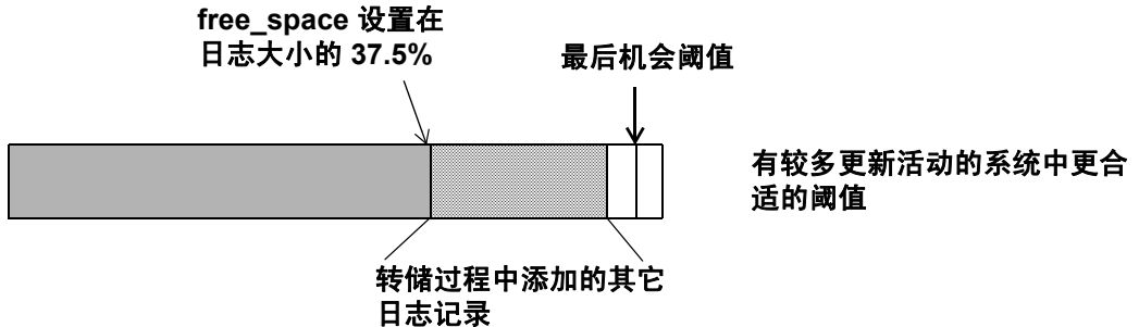
图 16-9：移动阈值以留下足够的可用空间来完成转储
