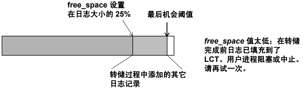
图 16-8：其它日志阈值未能及时开始转储
