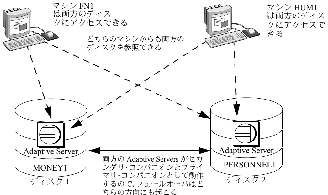
図 3-2: 高可用性システムにおける対称型設定
