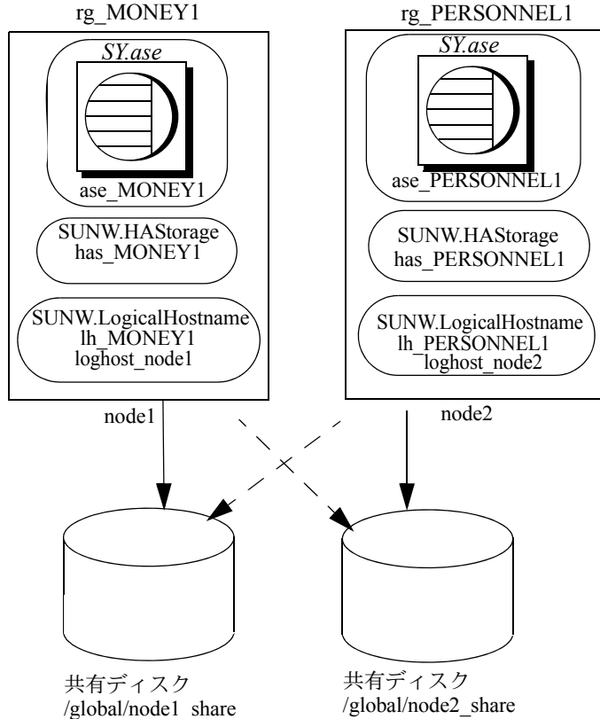
図 9-1: Sun Cluster リソース・グループの設定例
