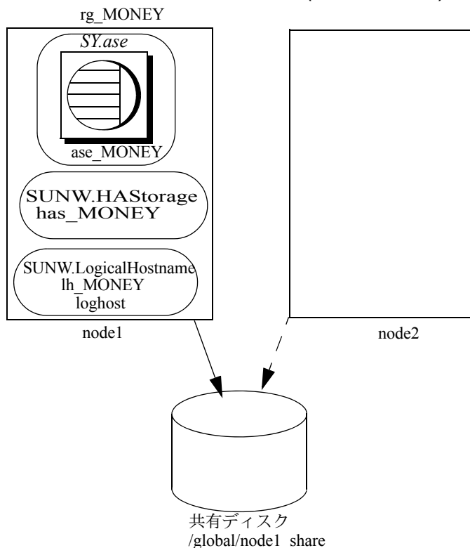
図 10-1: Sun Cluster のアクティブ/パッシブ設定 (フェールオーバー前)
