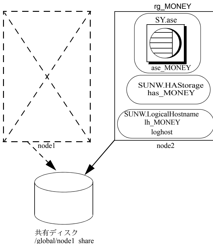
図 10-2: Sun Cluster のアクティブ/パッシブ設定 (フェールオーバー後)
