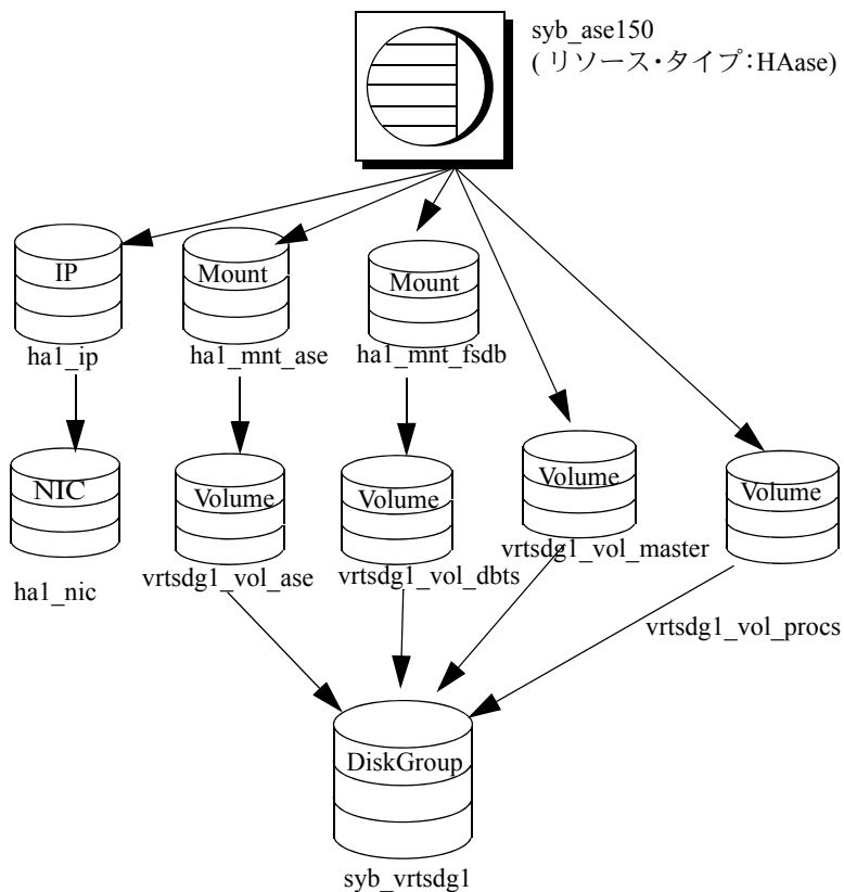
図 11-1: Veritas Cluster Server で動作するサービス・グループのサンプル
