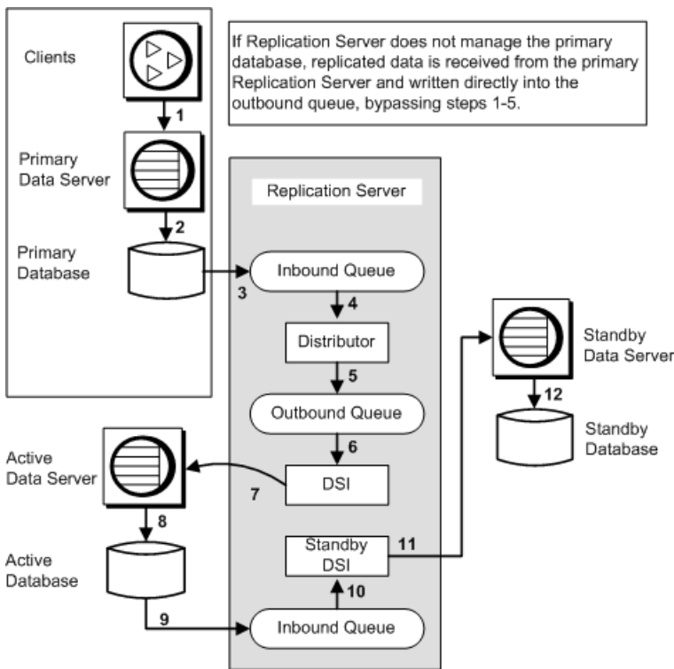
图 10： 复制数据库的热备份应用程序
