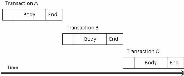
图 17: 使用 wait_after_commit 序列化方法的线程计时
