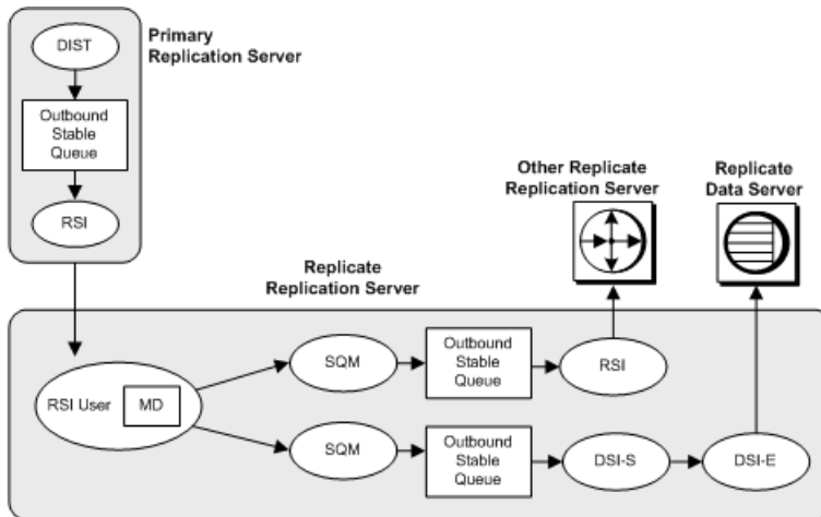
图 12: 复制 Replication Server 中的事务处理
