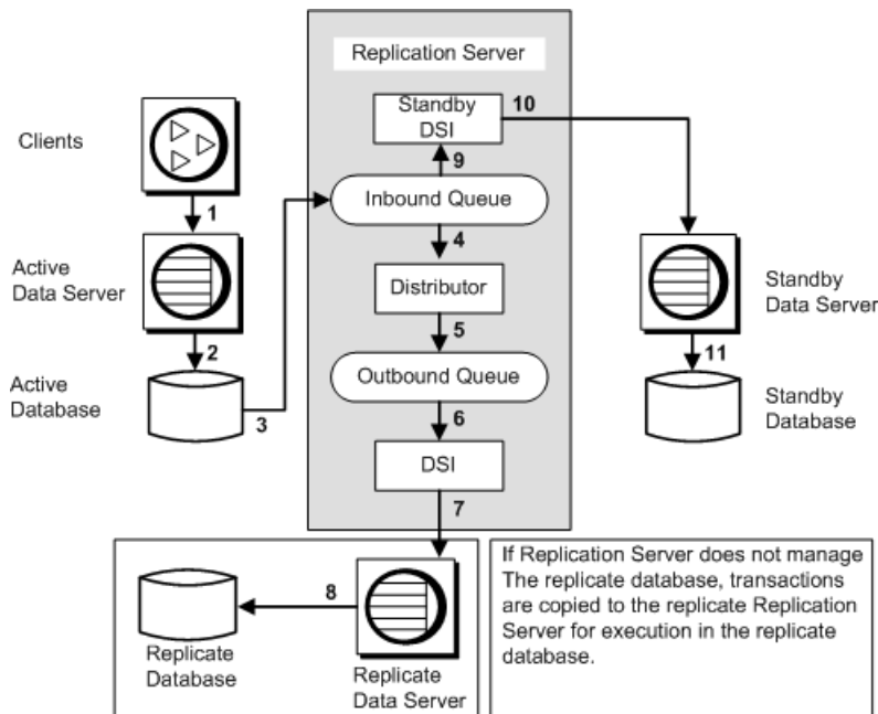
图 9：主数据库的热备份应用程序
