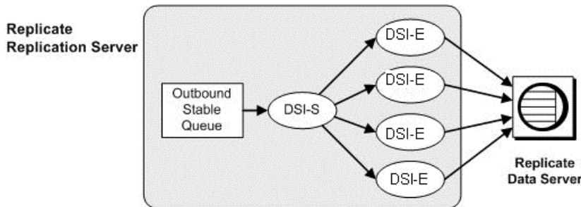
图 13：并行 DSI 的组件
