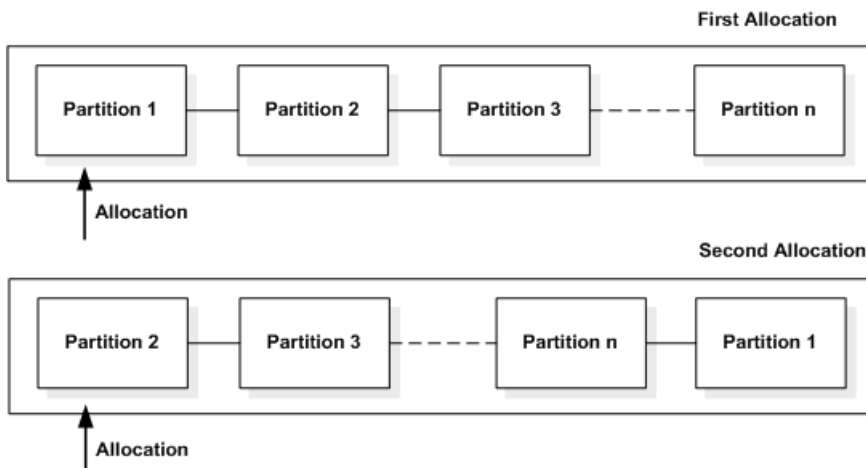
图 22：缺省分配机制
