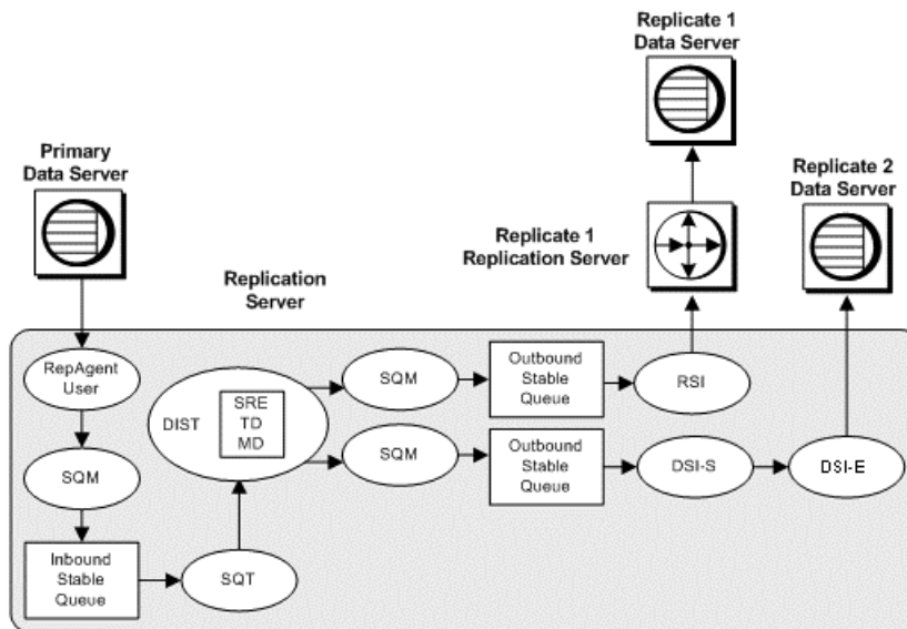
图 11：用于主 Replication Server 中的处理的线程
