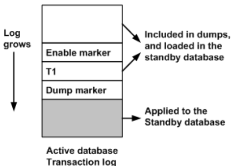
图 4：使用带有转储标记的 dump 和 load 命令
