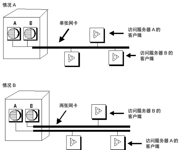
图 4-2：隔离重网络负荷用户
